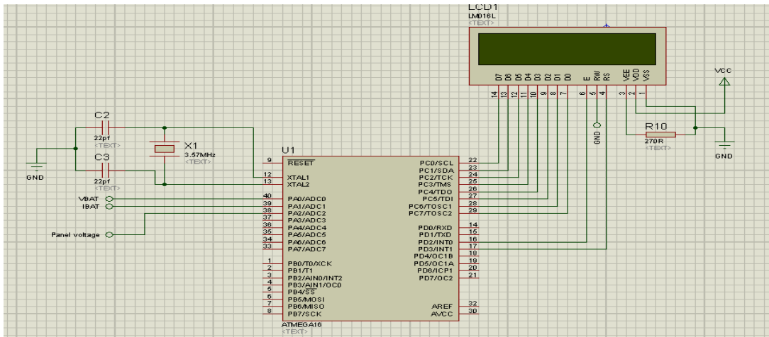
Fig. 2 AVR Microcontroller
